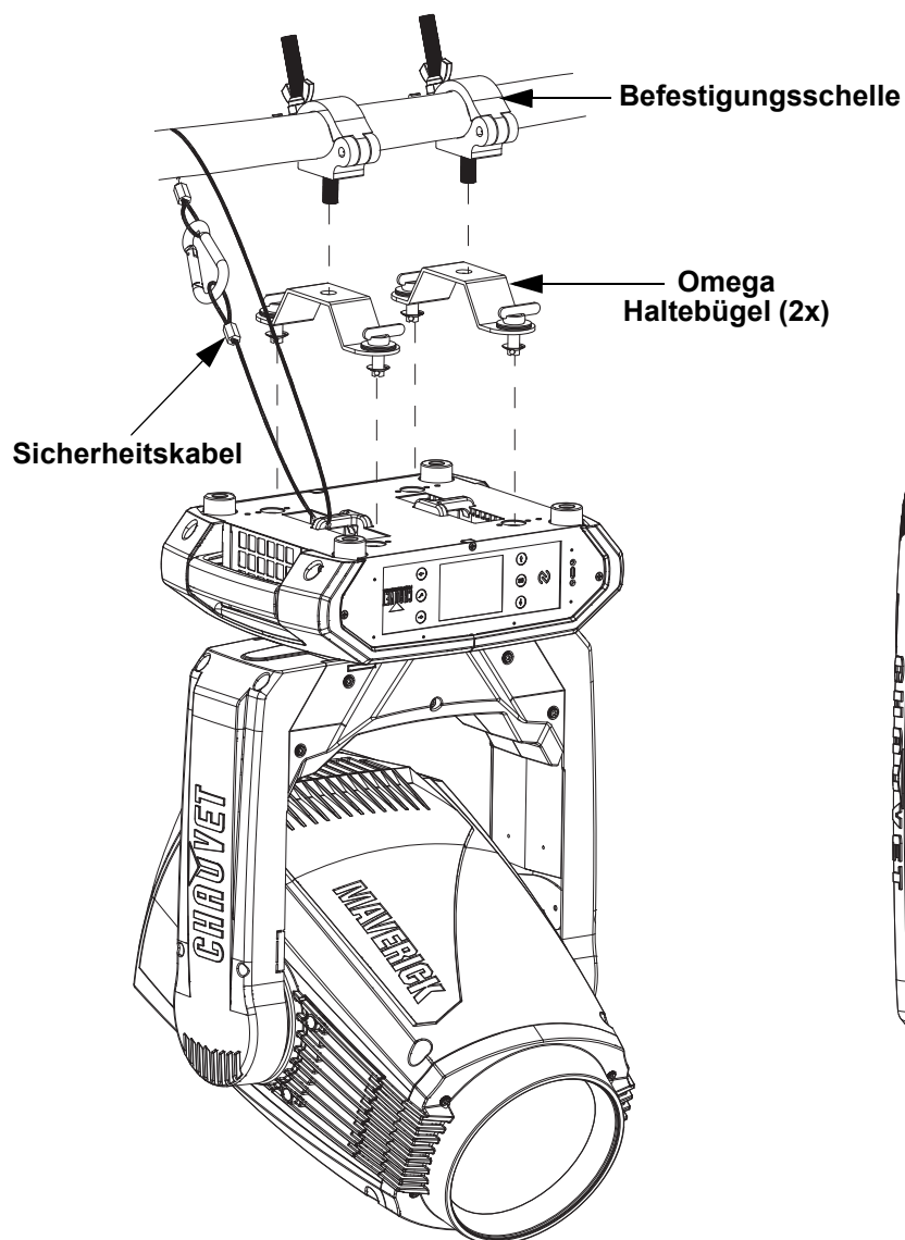
Montage über Kopf
