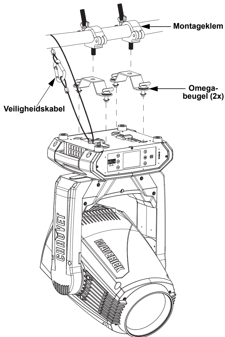
Montage boven het hoofd
