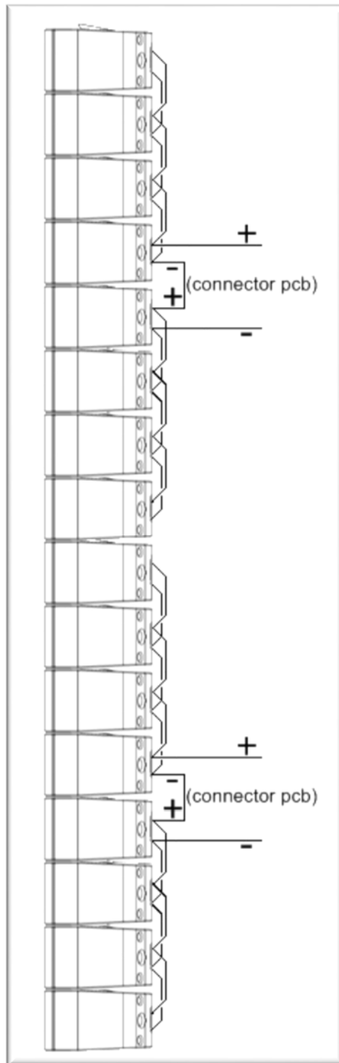
16 module array (8 ohms per channel)
