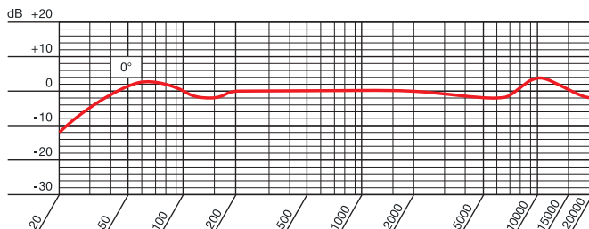
Frequenzkurve
