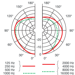
Polardiagramm
