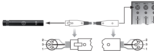
Abbildung 2: Anschluss an einen symmetrischen Eingang mit Phantomspeisung
