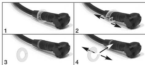
Fig. 3: Substituir o anel de gotejamento
