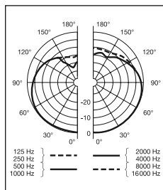
Polardiagramm
