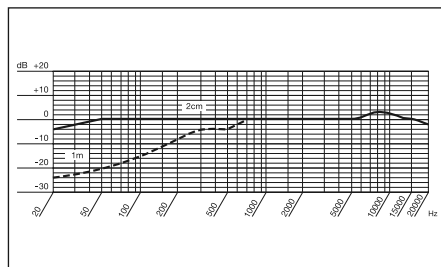
Frequenzkurve
